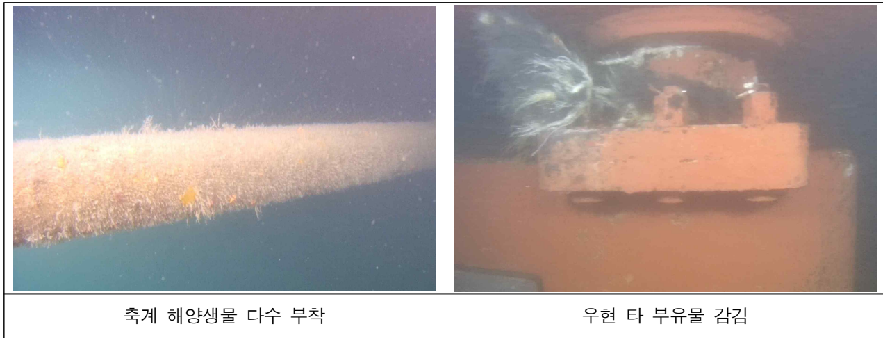
[사진 2] 관내·외 유도선 수면하부 점검 사진
