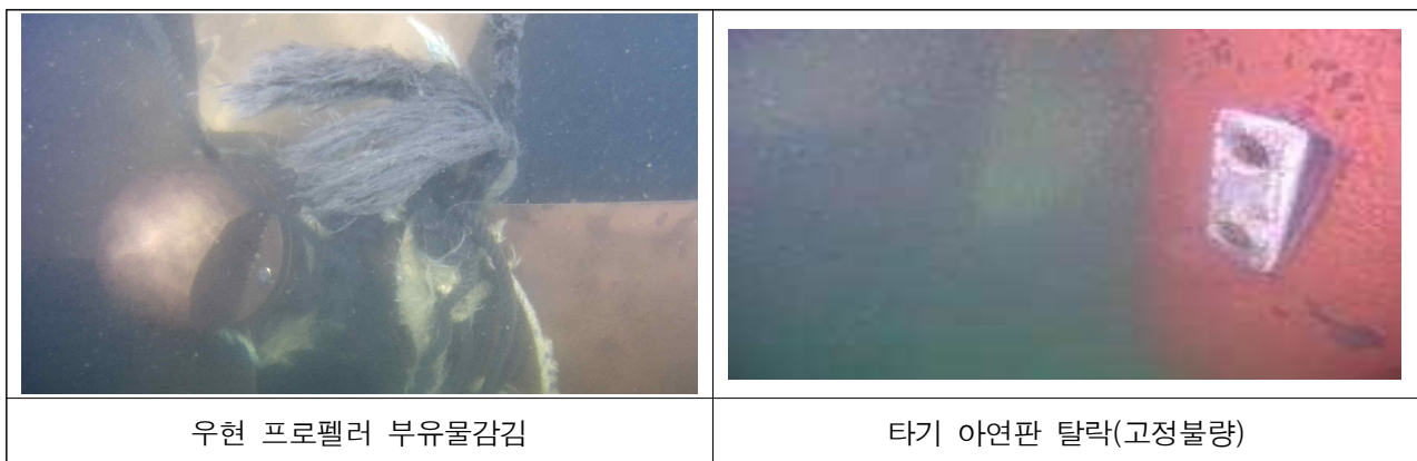
[사진 1] 관내 여객선 및 관공선 수면하부 점검 사진
